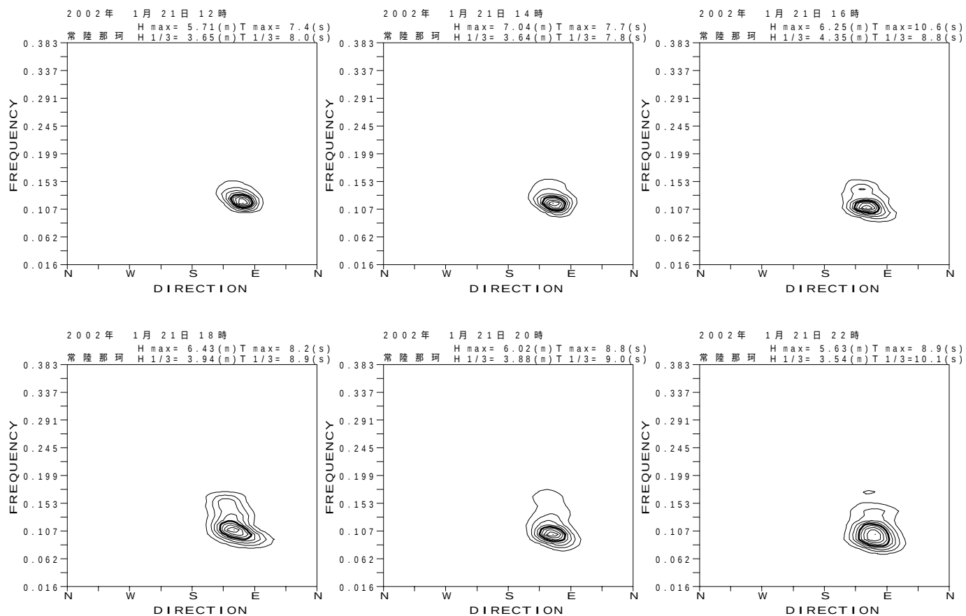
付図 - B.3.33 常陸那珂 代表的な高波期間中の方向スペクトル
