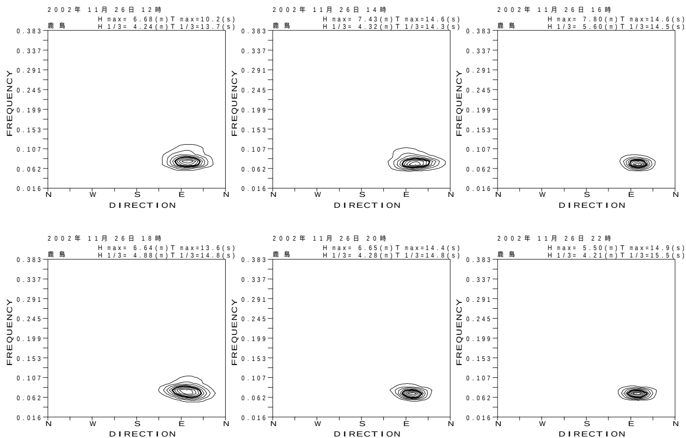
付図 - B.3.34 鹿島 代表的な高波期間中の方向スペクトル
