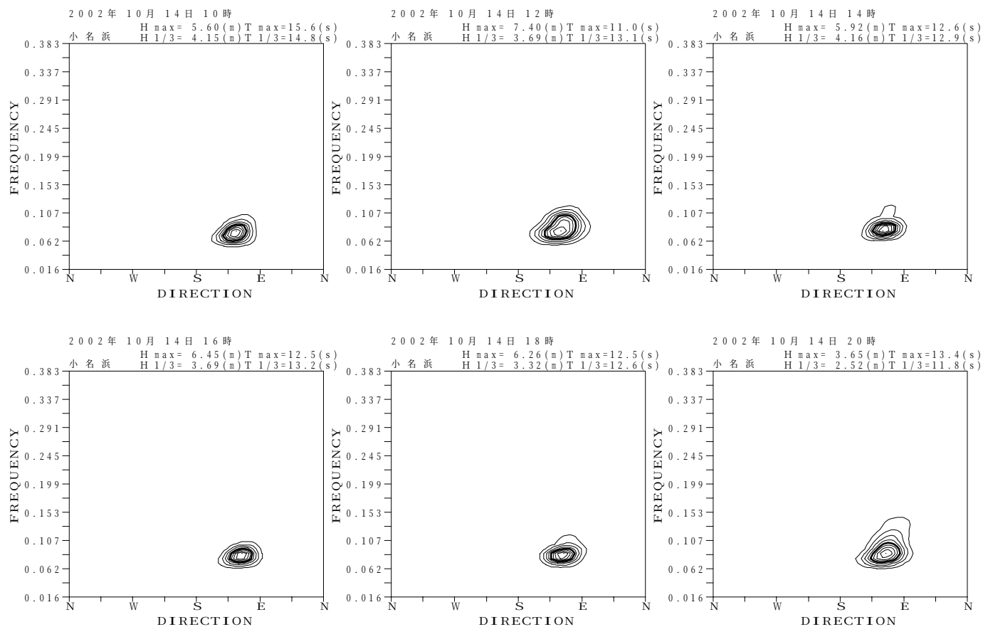
付図－B.3.32 小名浜 代表的な高波期間中の方向スペクトル
