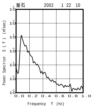
付図 - B.3.28 釜石 代表的な高波期間中のスペクトル
