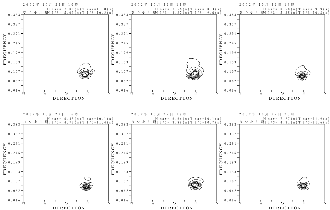
付図-B.3.25 むつ小川原 代表的な高波期間中の方向スペクトル
