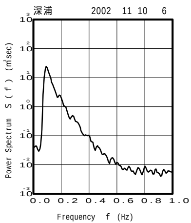
付図 - B.3.3 深浦 代表的な高波期間中のスペクトル
