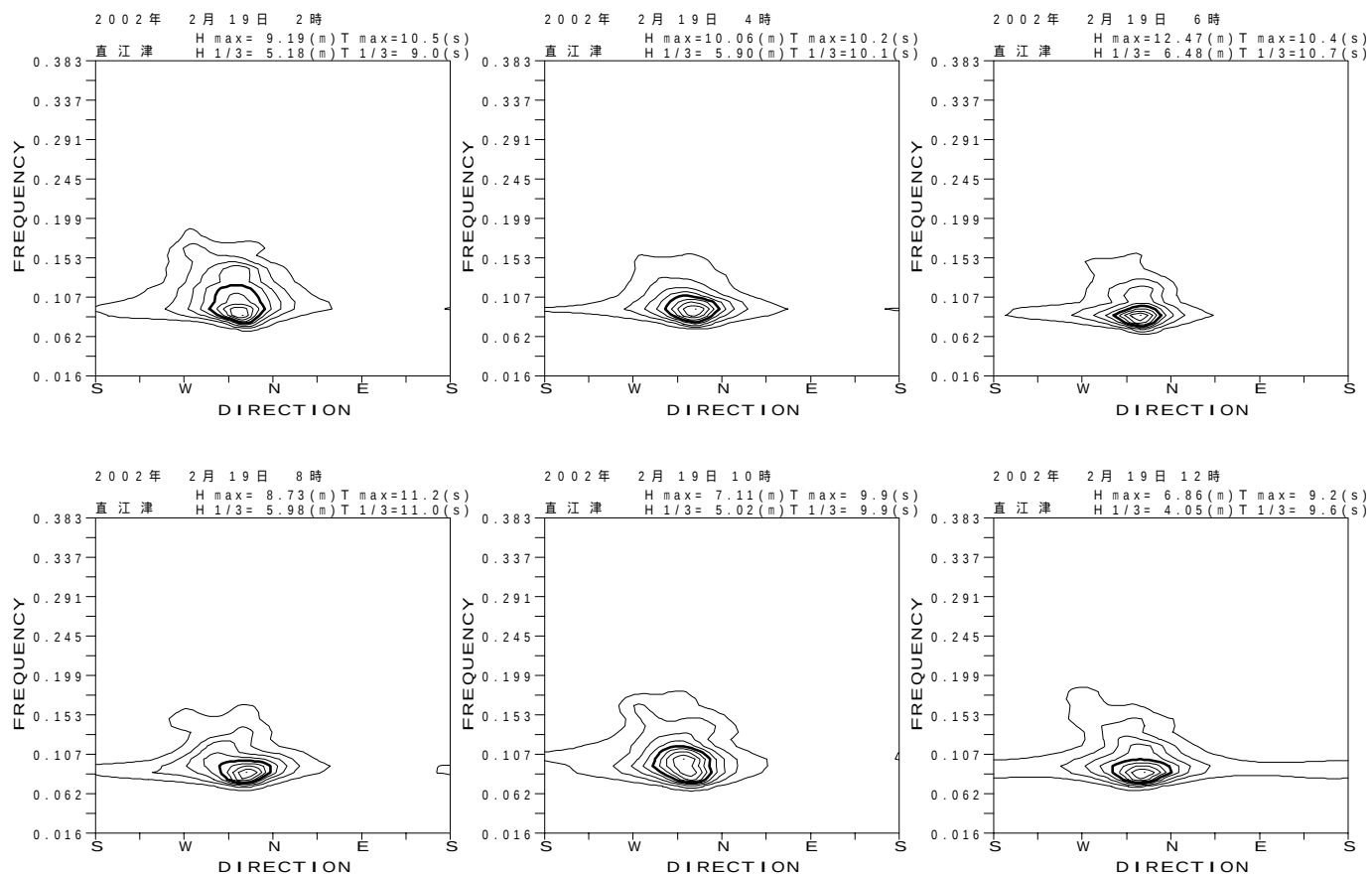
付図 - B.3.7 直江津 代表的な高波期間中の方向スペクトル
