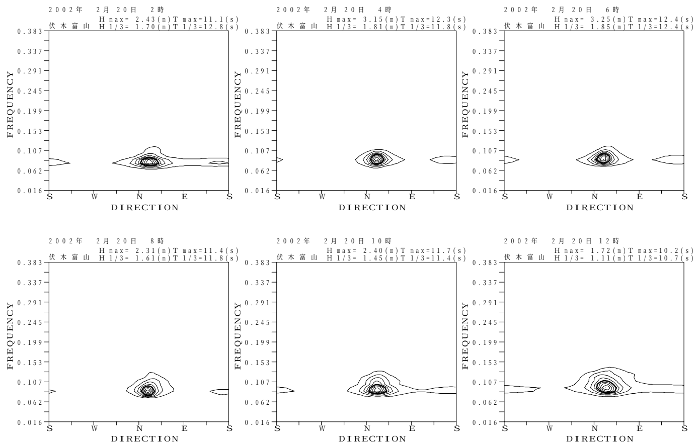
付図-B.3.9 伏木富山 代表的な高波期間中の方向スペクトル
