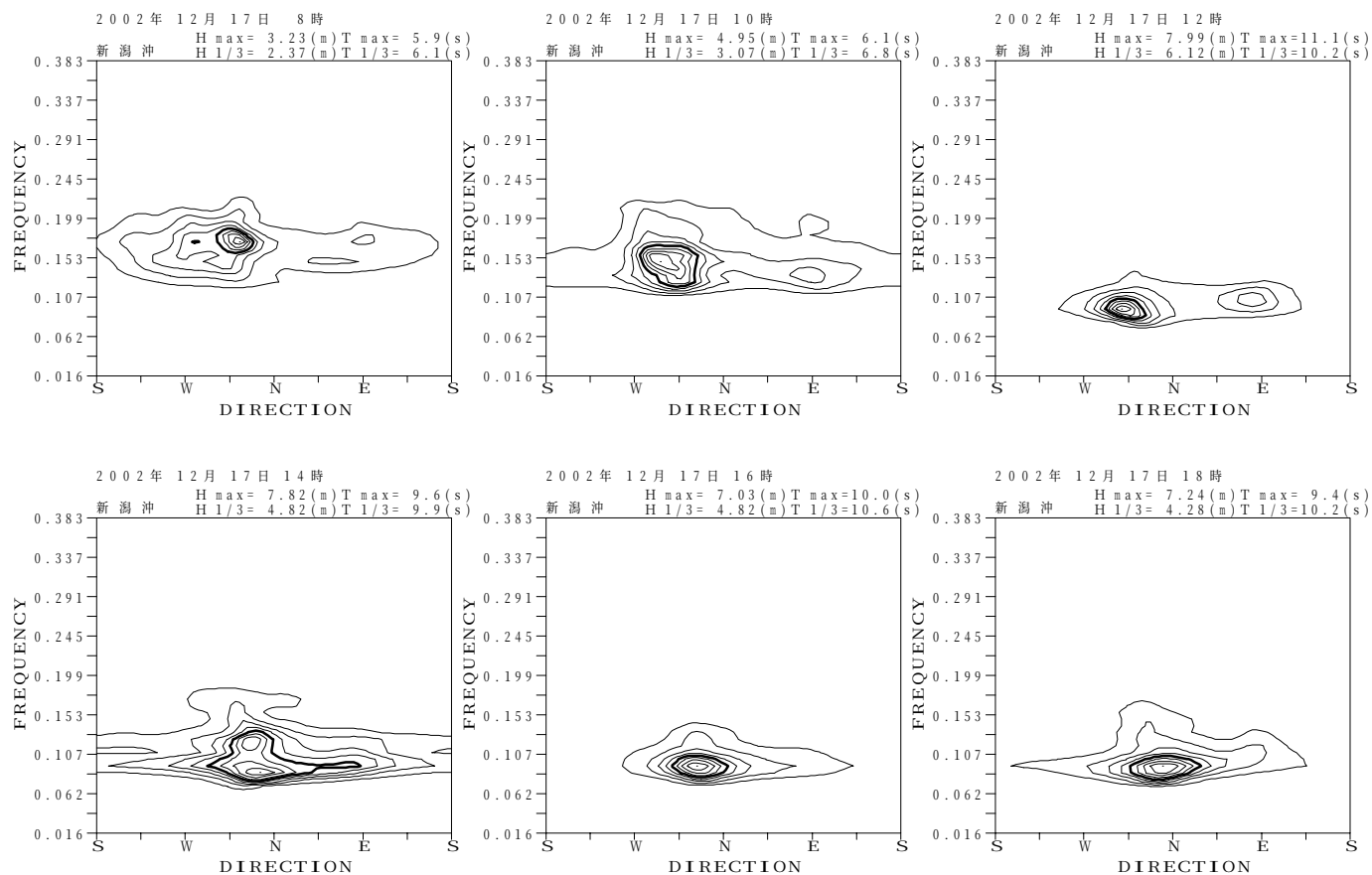
付図-B.3.6 新潟沖 代表的な高波期間中の方向スペクトル
