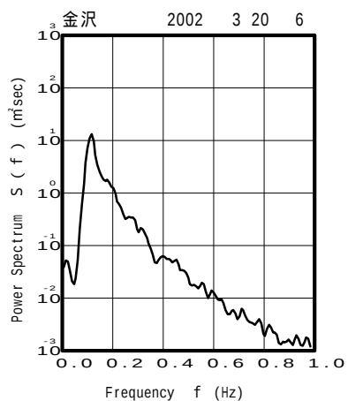
付図 - B.3.11 金沢 代表的な高波期間中のスペクトル
