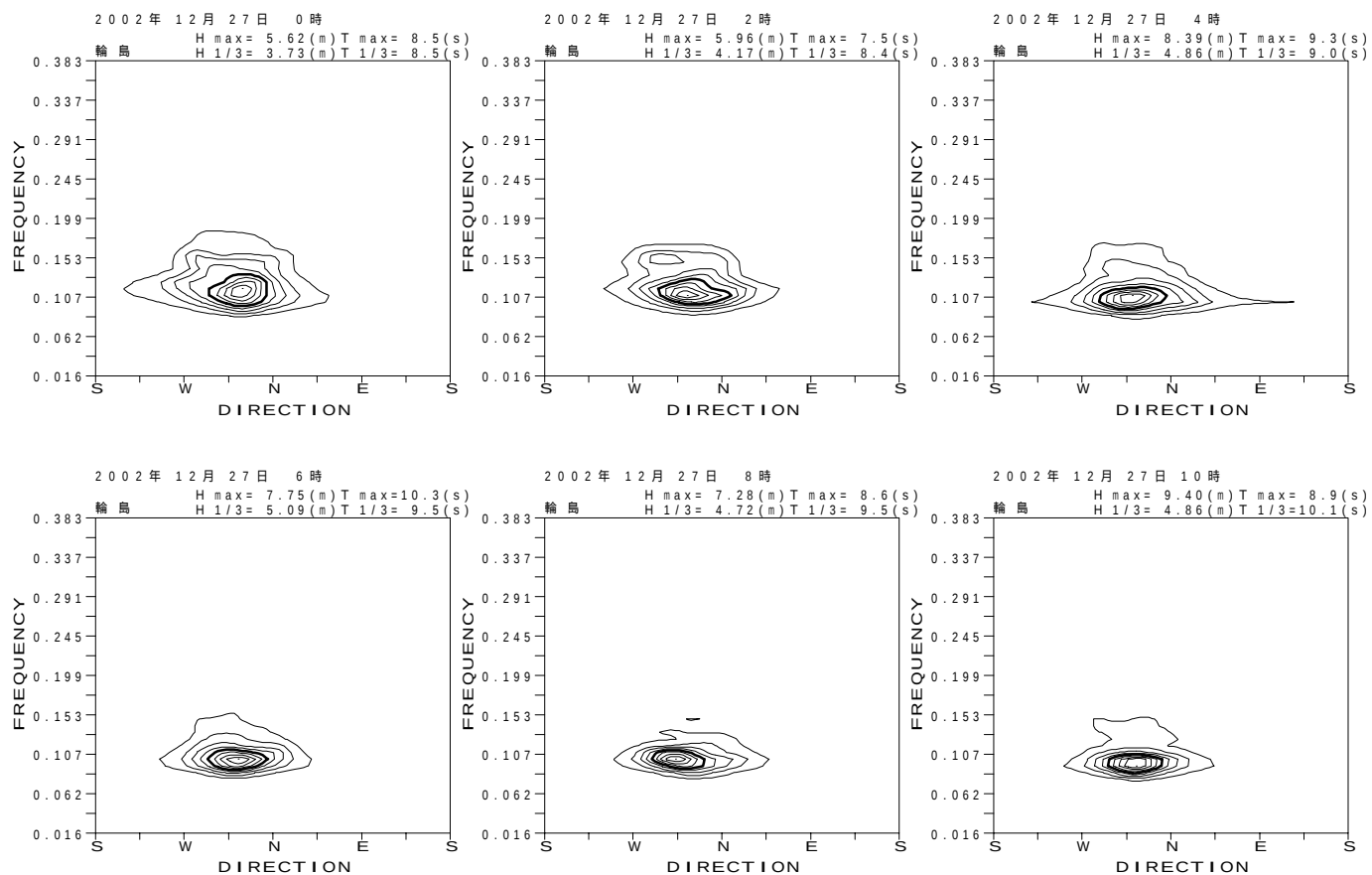
付図 - B.3.10 輪島 代表的な高波期間中の方向スペクトル
