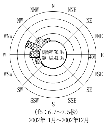
付図-B.2.2 瀬棚 波高・波向別出現頻度図 (f2, f3, f4, f5, 全周期帯)
