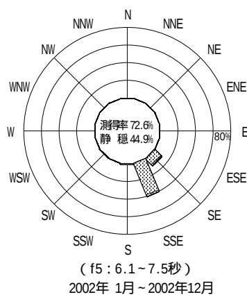
付図 - B.2.24 苫小牧 波高・波向別出現頻度図 ( f2 , f3 , f4 , f5 , 全周期帯 )
