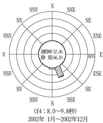
付図-B.2.39 清水 波高・波向別出現頻度図 (f2, f3, f4, f5, 全周期帯)
