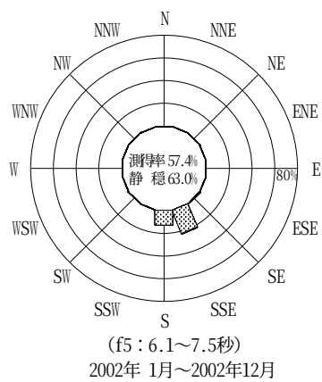
付図-B.2.39 清水 波高・波向別出現頻度図 (f2, f3, f4, f5, 全周期帯)
