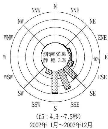
付図-B.2.40 御前崎 波高・波向別出現頻度図 (f2, f3, f4, f5, 全周期帯)
