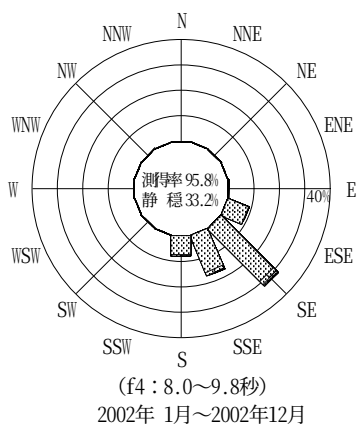
付図-B.2.40 御前崎 波高・波向別出現頻度図 (f2, f3, f4, f5, 全周期帯)
