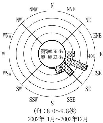
付図-B.2.49 細島 波高・波向別出現頻度図 (f2, f3, f4, f5, 全周期帯)
