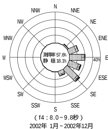
付図 - B.2.50 宮崎 波高・波向別出現頻度図 ( f2 , f3 , f4 , f5 , 全周期帯 )
