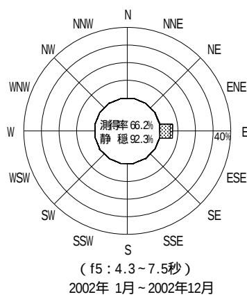
付図 - B.2.48 苅田 波高・波向別出現頻度図 ( f2 , f3 , f4 , f5 , 全周期帯 )
