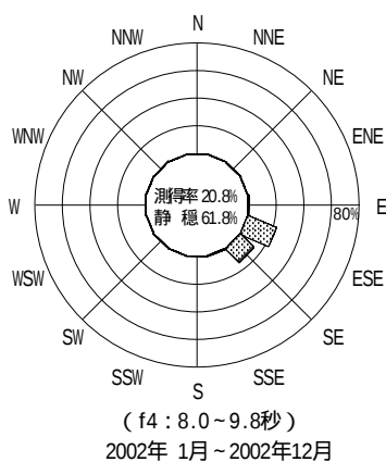
付図 - B.2.51 志布志湾 波高・波向別出現頻度図 ( f2 , f3 , f4 , f5 , 全周期帯 )
