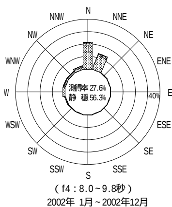
付図 - B.2.18 玄界灘 波高・波向別出現頻度図 ( f2 , f3 , f4 , f5 , 全周期帯 )
