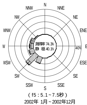
付図 - B.2.19 伊王島 波高・波向別出現頻度図 ( f2 , f3 , f4 , f5 , 全周期帯 )
