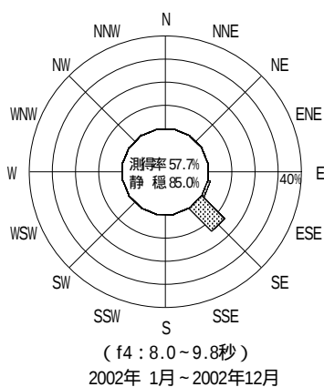
付図 - B.2.44 小松島 波高・波向別出現頻度図 ( f2 , f3 , f4 , f5 , 全周期帯 )
