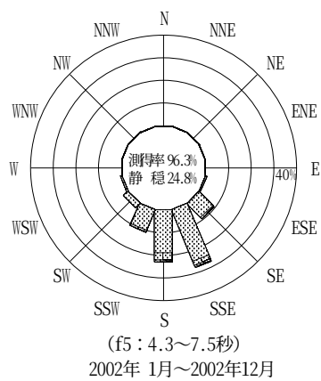
付図-B.2.46 高知 波高・波向別出現頻度図 (f2, f3, f4, f5, 全周期帯)
