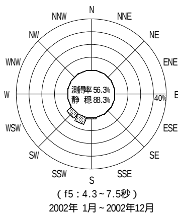
付図 - B.2.43 神戸 波高・波向別出現頻度図 ( f2 , f3 , f4 , f5 , 全周期帯 )
