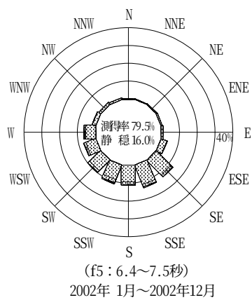
付図-B.2.42 潮岬 波高・波向別出現頻度図 (f2, f3, f4, f5, 全周期帯)
