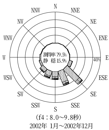
付図-B.2.42 潮岬 波高・波向別出現頻度図 (f2, f3, f4, f5, 全周期帯)
