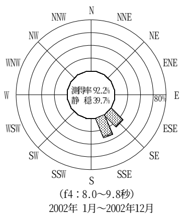
付図-B.2.29 石巻 波高・波向別出現頻度図 (f2, f3, f4, f5, 全周期帯)
