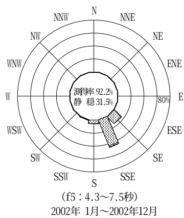
付図-B.2.29 石巻 波高・波向別出現頻度図 (f2, f3, f4, f5, 全周期帯)
