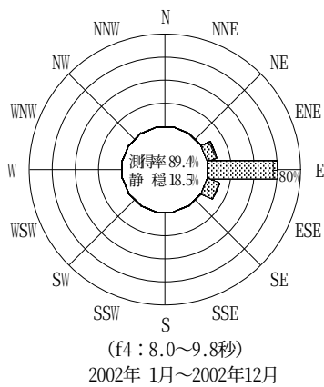
付図-B.2.31 相馬 波高・波向別出現頻度図 (f2, f3, f4, f5, 全周期帯)
