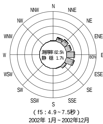
付図 - B.2.33 常陸那珂 波高・波向別出現頻度図 ( f2 , f3 , f4 , f5 , 全周期帯 )
