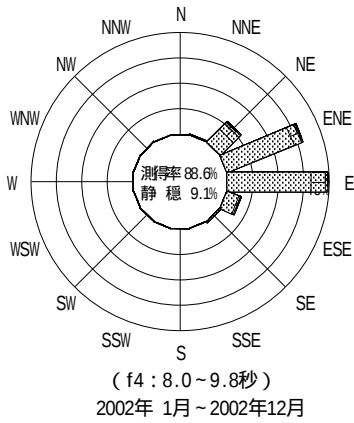
付図 - B.2.34 鹿島 波高・波向別出現頻度図 ( f2 , f3 , f4 , f5 , 全周期帯 )
