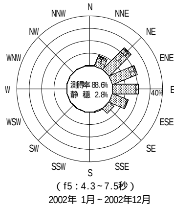
付図 - B.2.34 鹿島 波高・波向別出現頻度図 ( f2 , f3 , f4 , f5 , 全周期帯 )
