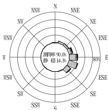
付図-B.2.25 むつ小川原 波高・波向別出現頻度図 (f2, f3, f4, f5, 全周期帯)
