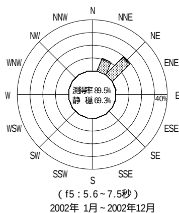
付図 - B.2.9 伏木富山 波高・波向別出現頻度図 ( f2 , f3 , f4 , f5 , 全周期帯 )
