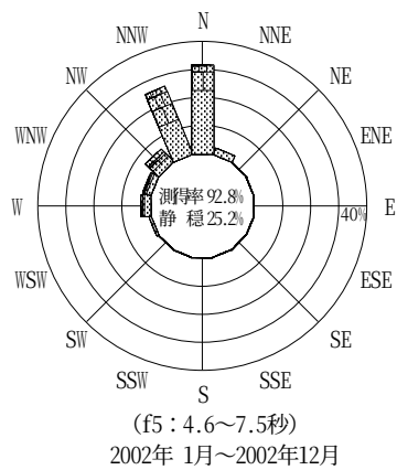
付図-B.2.6 新潟沖 波高・波向別出現頻度図 (f2, f3, f4, f5, 全周期帯)
