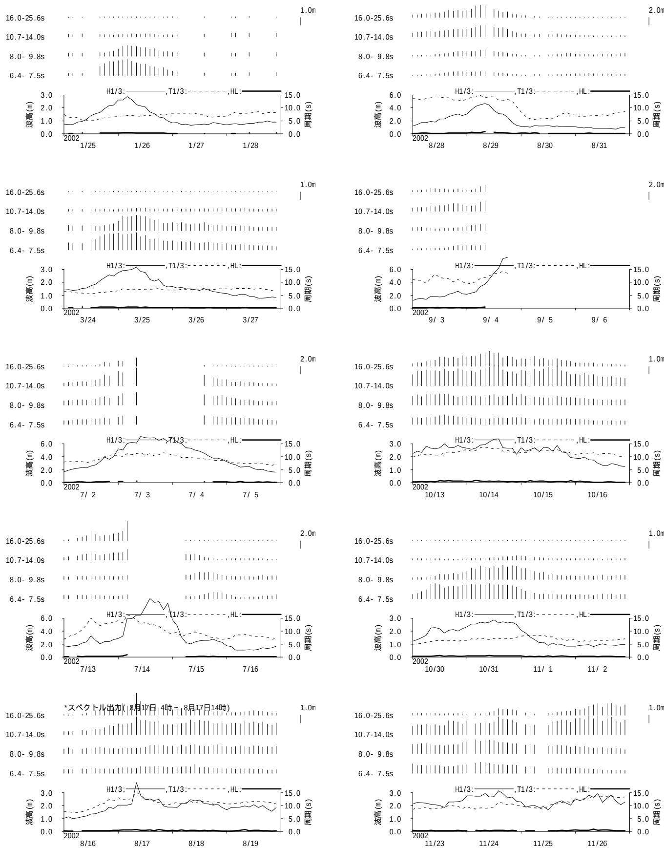
付図 - B.1.53 中城湾 周期帯別波浪特性の経時変化(高波期間中)
