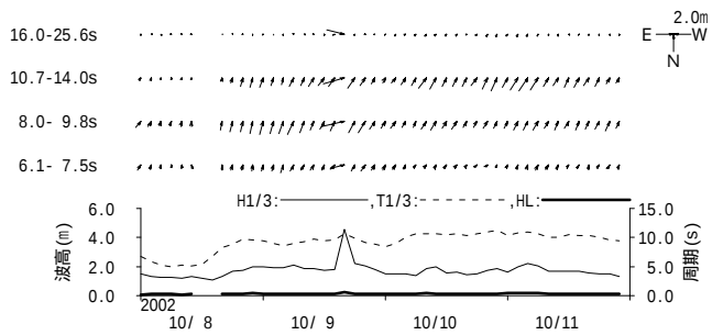
付図 - B.1.22 紋別(南) 周期帯別波浪特性の経時変化(高波期間中)
