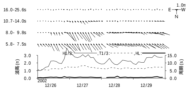
付図 - B.1.1 留萌 周期帯別波浪特性の経時変化(高波期間中)
