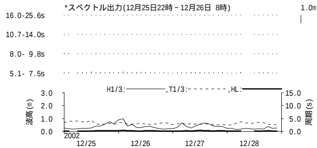
付図 - B.1.41 伊勢湾 周期帯別波浪特性の経時変化(高波期間中)
