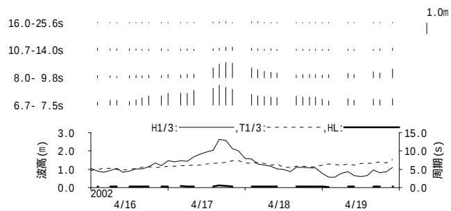
付図 - B.1.38 下田 周期帯別波浪特性の経時変化(高波期間中)
