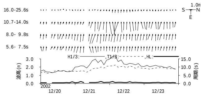
付図 - B.1.49 細島 周期帯別波浪特性の経時変化(高波期間中)
