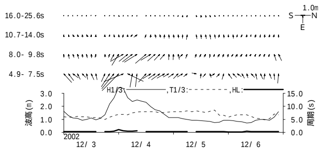
付図 - B.1.50 宮崎 周期帯別波浪特性の経時変化(高波期間中)
