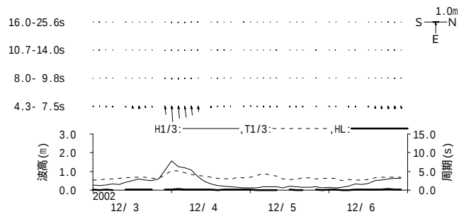
付図 - B.1.48 苅田 周期帯別波浪特性の経時変化(高波期間中)
