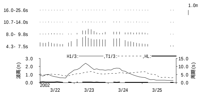
付図 - B.1.17 藍島 周期帯別波浪特性の経時変化(高波期間中)
