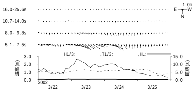
付図 - B.1.18 玄界灘 周期帯別波浪特性の経時変化(高波期間中)
