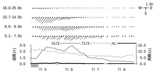
付図 - B.1.19 伊王島 周期帯別波浪特性の経時変化(高波期間中)
