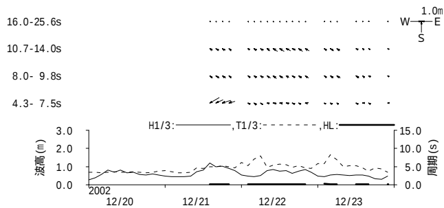
付図 - B.1.44 小松島 周期帯別波浪特性の経時変化(高波期間中)
