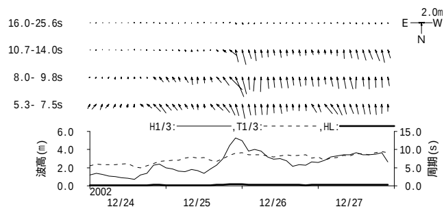
付図 - B.1.12 柴山 周期帯別波浪特性の経時変化(高波期間中)
