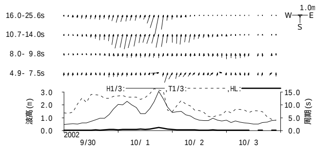
付図 - B.1.45 室津 周期帯別波浪特性の経時変化(高波期間中)
