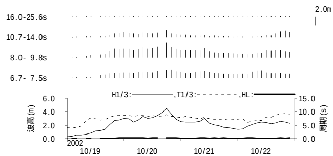
付図 - B.1.16 浜田 周期帯別波浪特性の経時変化(高波期間中)
