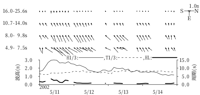
付図-B.1.33 常陸那珂 周期帯別波浪特性の経時変化(高波期間中)
