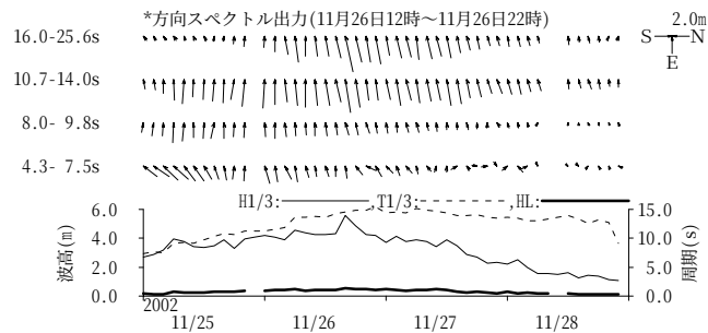
付図-B.1.34 鹿島 周期帯別波浪特性の経時変化(高波期間中)
