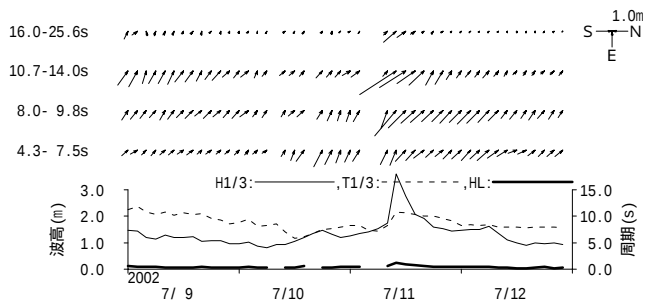
付図 - B.1.30 仙台新港 周期帯別波浪特性の経時変化(高波期間中)
